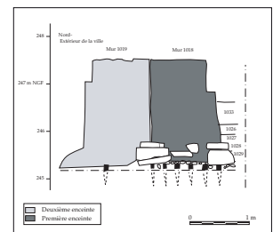
Fig. 3 : Sarrebourg (57), Coupe des courtines soutenues par des fondations sur pieux (DAO : N. Meyer / INRAP)
